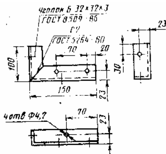
Уголок (поз.4)
