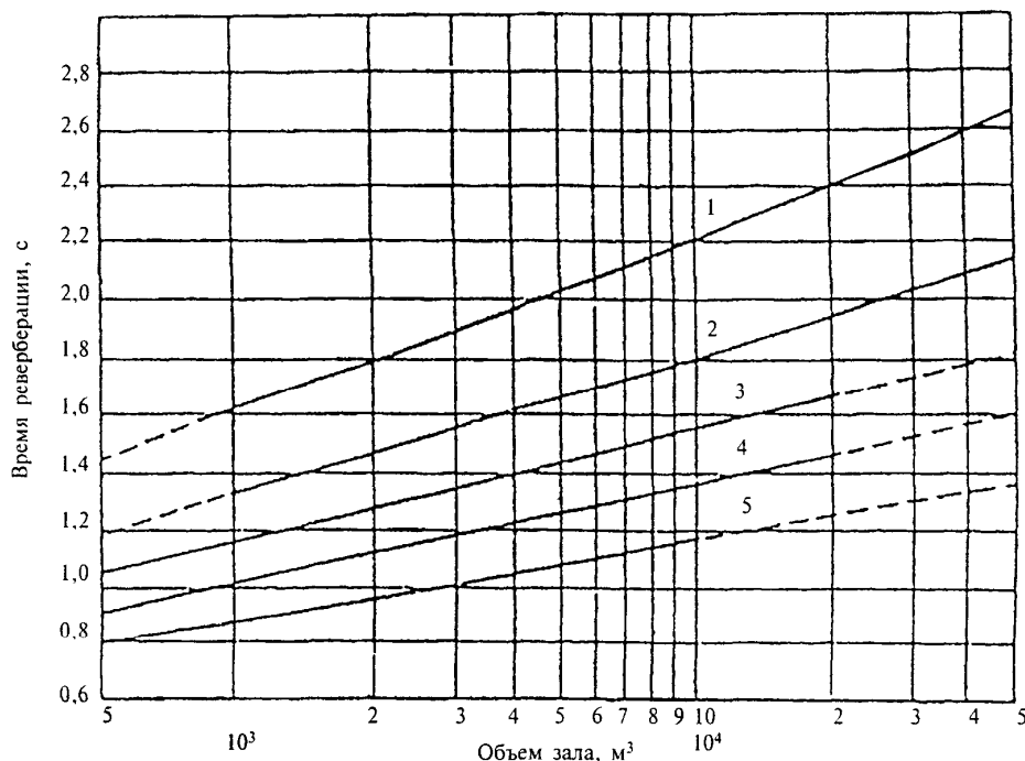
Рисунок 6 — Рекомендуемое время реверберации на средних частотах (500—1000 Гц) для залов различного назначения в зависимости от их объема
