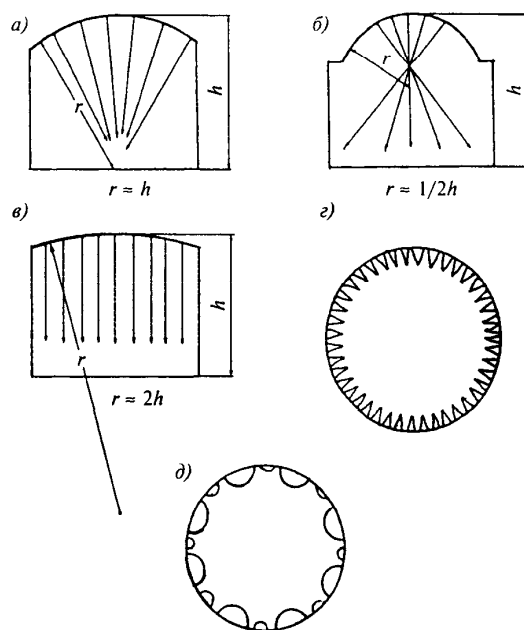
Рисунок 9 — Варианты решения зала с куполом
