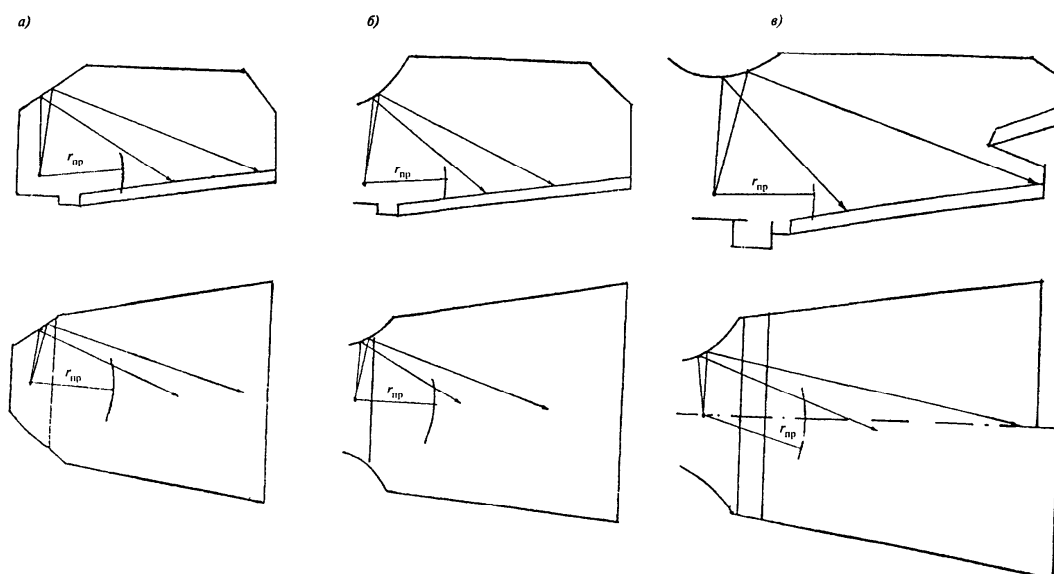
Рисунок 7 — Оформление портала, позволяющее направить первые отражения в глубину зала
