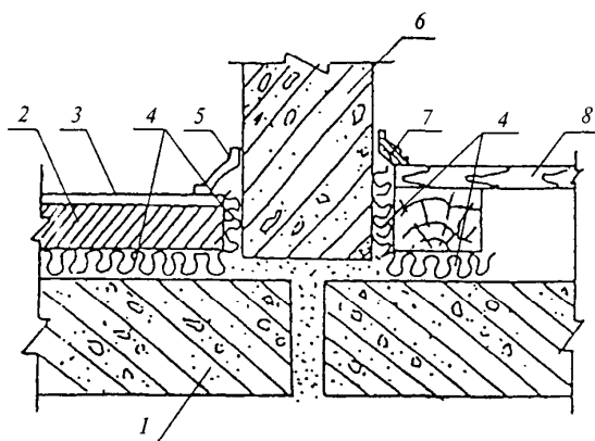
1 — несущая часть междуэтажного перекрытия; 2 — бетонное основание пола; 3 — покрытие пола; 4 — прокладка (слой) из звукоизоляционного материала; 5 — гибкий пластмассовый плинтус; 6 — стена; 7 — деревянная галтель; 8 — дощатый пол на лагах
