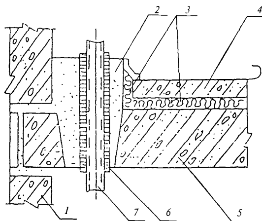
1 — стена; 2 — безусадочный бетон или раствор; 3 — прокладка (слой) из звукоизоляционного материала; 4 — бетонное основание пола; 5 — несущая часть перекрытия; 6 — эластичная гильза; 7 — труба стояка отопления
