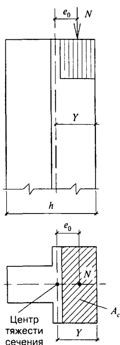
Рис. 5. Внецентренное сжатие
