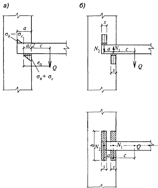
Рис. 14. Расчетные схемы заделки консольных балок
