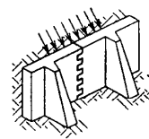
Рис. 3. Растяжение кладки при изгибе по перевязанному сечению
