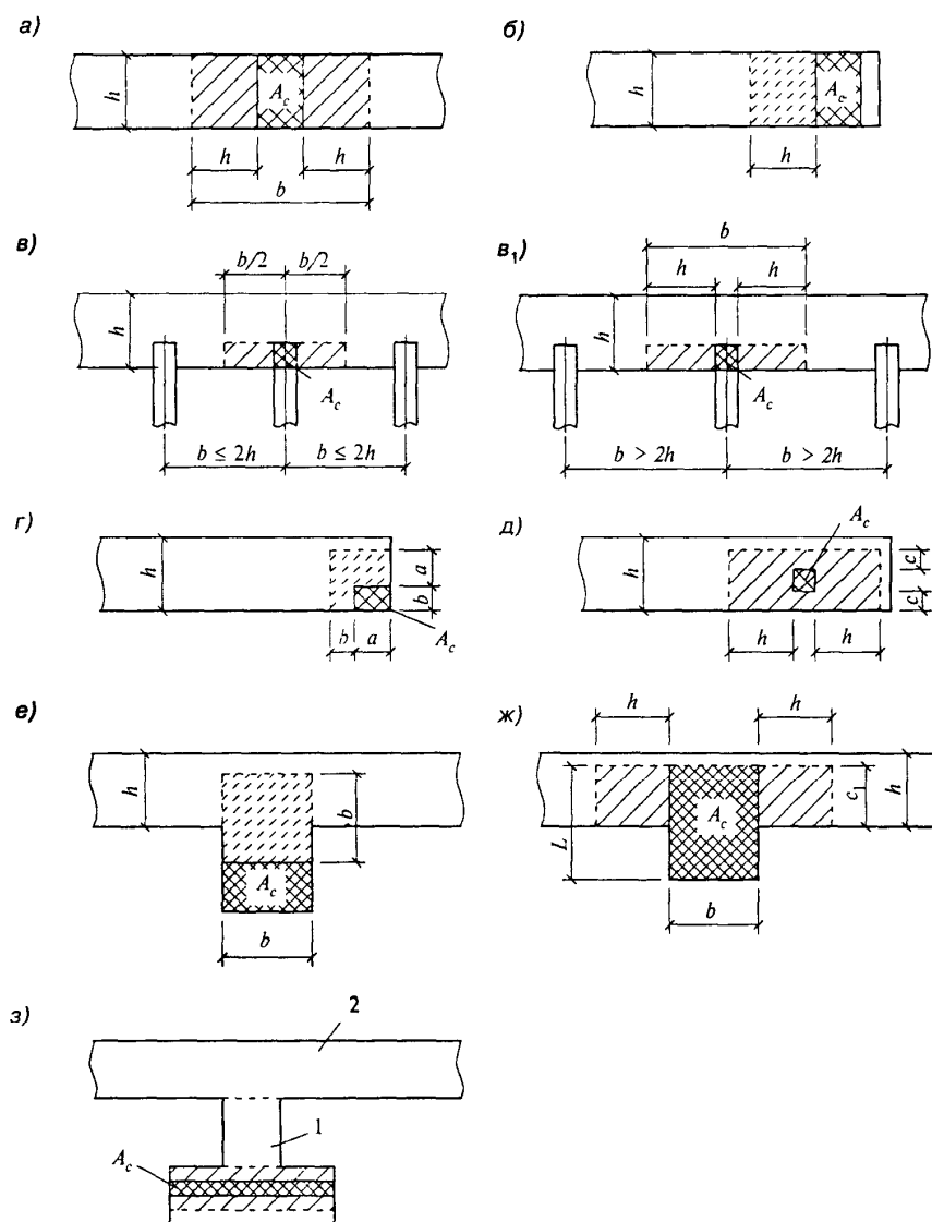
Рис. 9. Определение расчетных площадей сечений при местном сжатии
