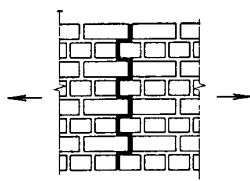
Рис. 2. Растяжение кладки по перевязанному сечению
